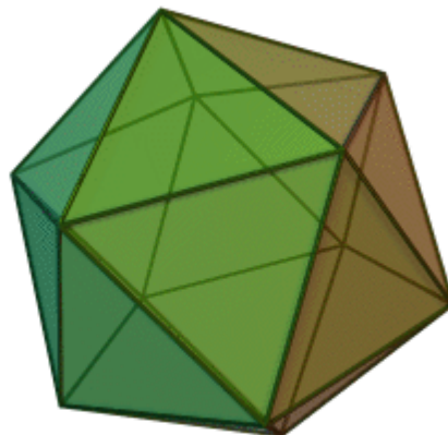
正二十面体
