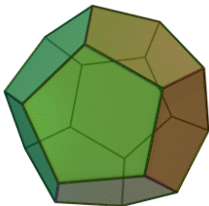
正十二面体
