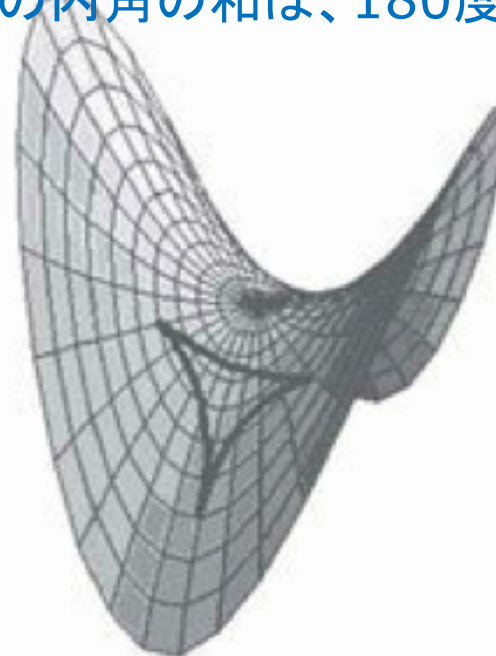
双曲幾何学
