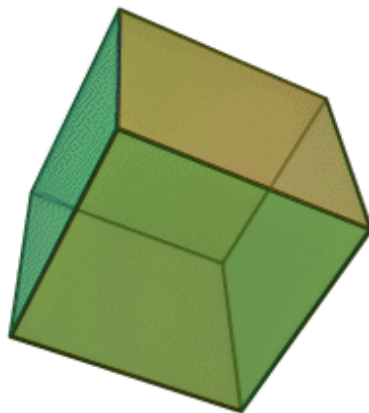
正六面体
